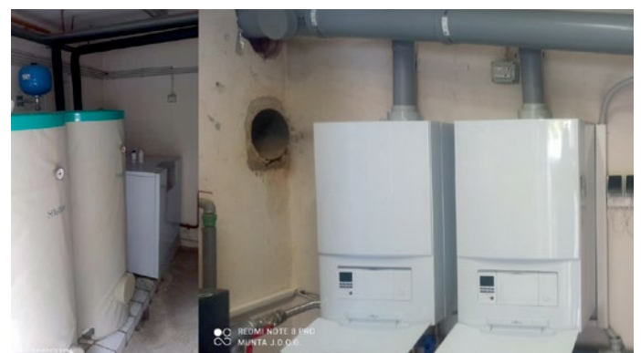
Stari atmoCRAFT i zamjena ecoTEC VU 486/5-5
