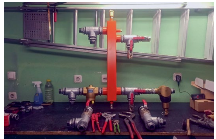
Sastavljanje sklopa u miru svoje radionice
