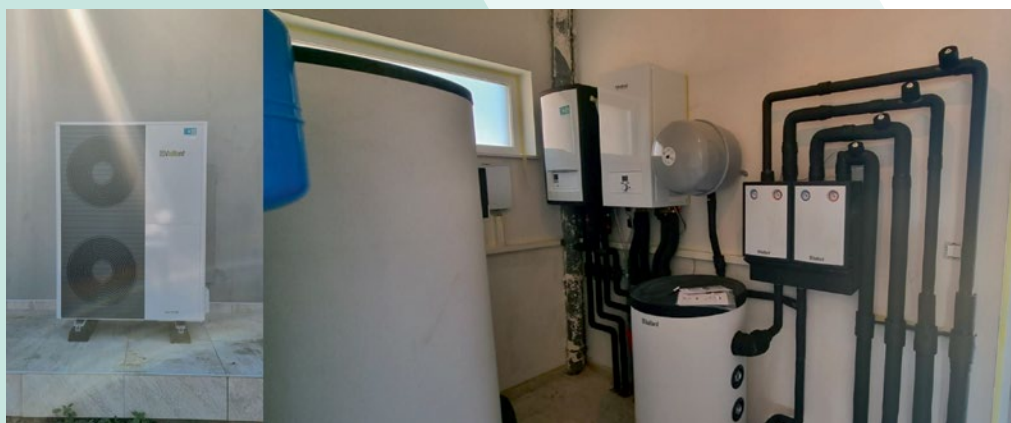
Dizalica topline aroTHERM VWL 125 s uređajem eloBLOCK 9 u Oprisavcima
