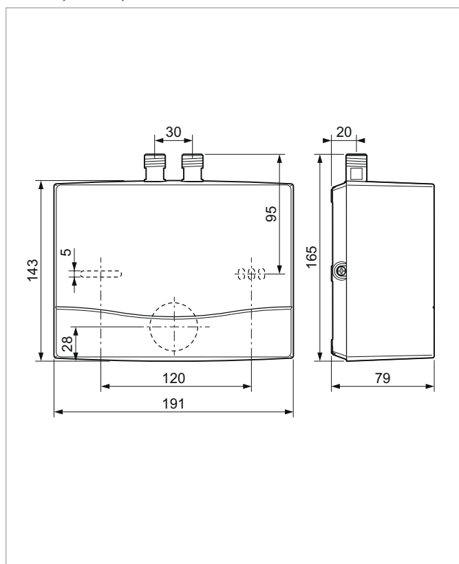
Dimenzije uređaja - miniVED
