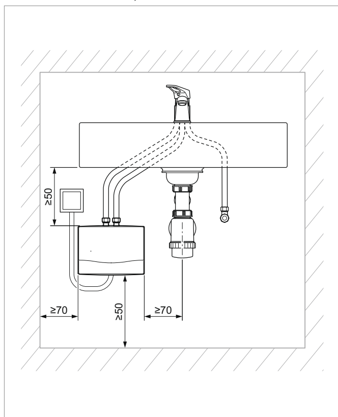
Minimalni razmaci uređaja - mini VED
